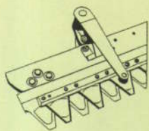
Doppel-Messerbalken Fingerbalken (ohne Bild)
